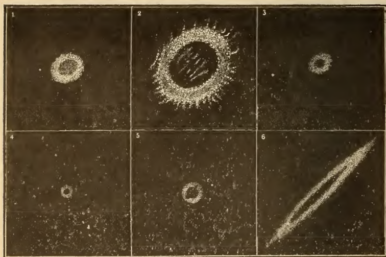
Annular Nebulae.
