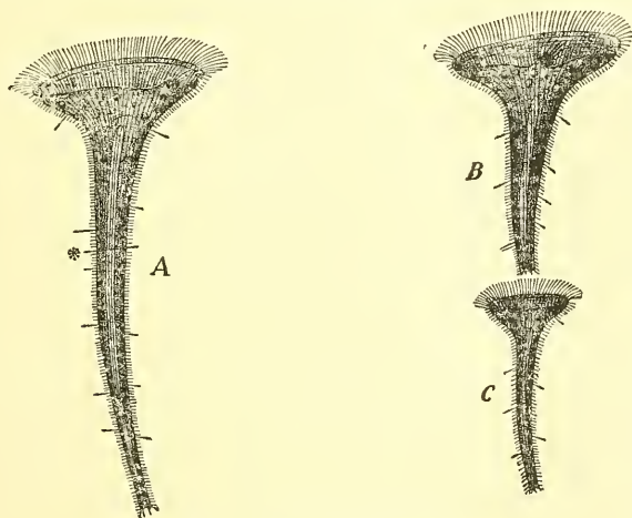
FIG. 6.— Stentor Roeselii .
