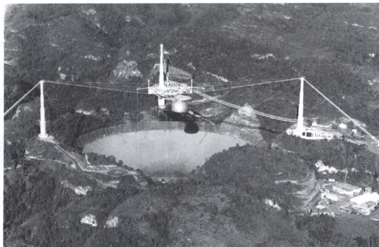
Verdens mest følsomme radioteleskop, Arecibo-teleskopet, på Puerto Rico. Reflektor-skålen har en diameter på 305 meter.
