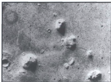
Det berømte Mars-ansigt ses her fotograferet af den amerikanske rumsonde Viking 1.
