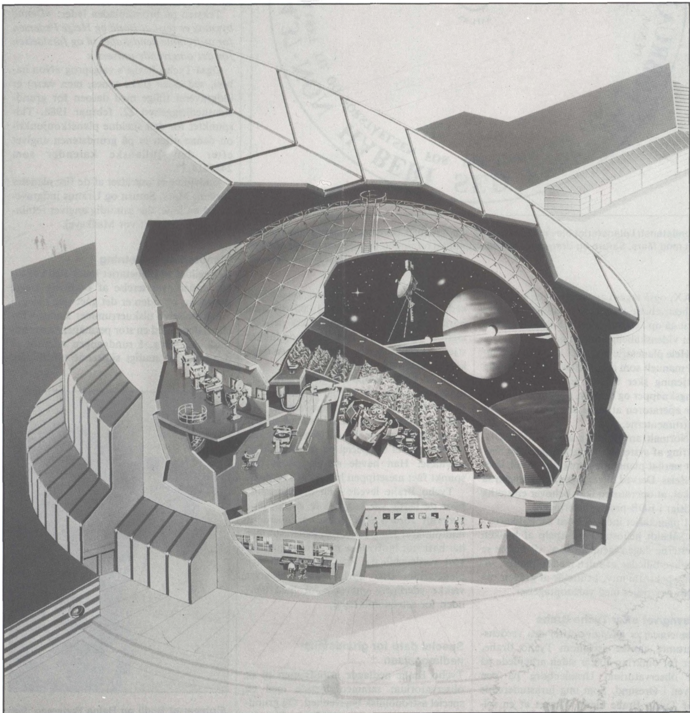
Tilskuerrummet og planetariekuppen med dens mange forskelligartede projektorer ses midt i tegningen over den specielle bygning. I stueetagen er der indrettet udstillings- og administrationslokaler samt restaurant.
