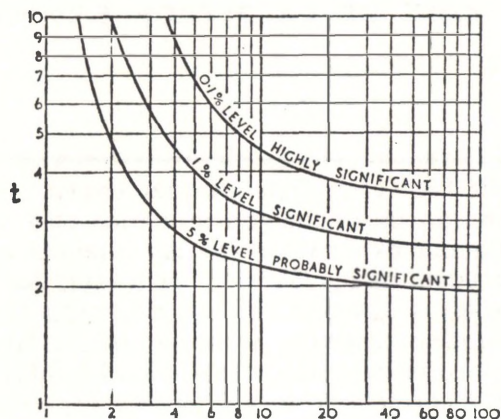
Figura 1 Gráfico t Student para los niveles de significación del 5%, 1%, y 0,1
