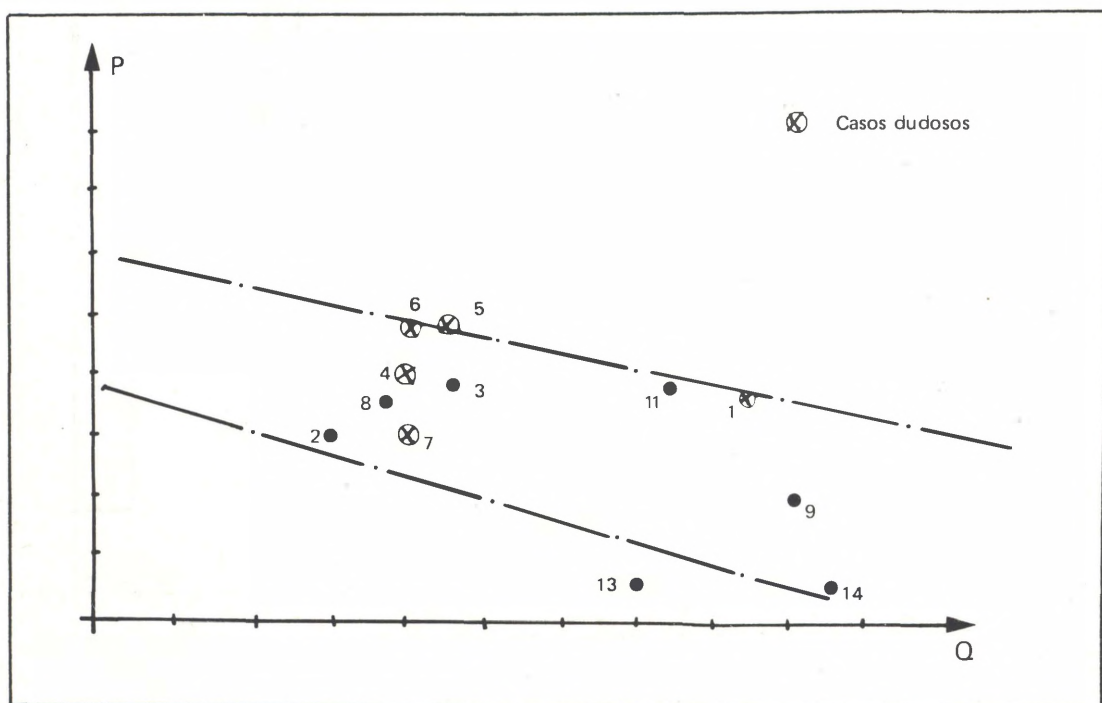
FIGURA 2. Clave: eje P = distribución de variaciones totales en el campo magnético terrestre durante tres horas antes y después de la observación de un OVNI; el eje Q = distancia en km del OVNI desde Chambon-la-Foret.
