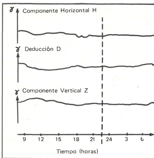
FIGURA 1. Grabación típica del magnetismo terrestre durante la observación de un OVNI. La línea de puntos representa el tiempo de la observación, que fue a una distancia de 58 km y sucedió el 24 de mayo de 1954, a las 22:15 horas.
