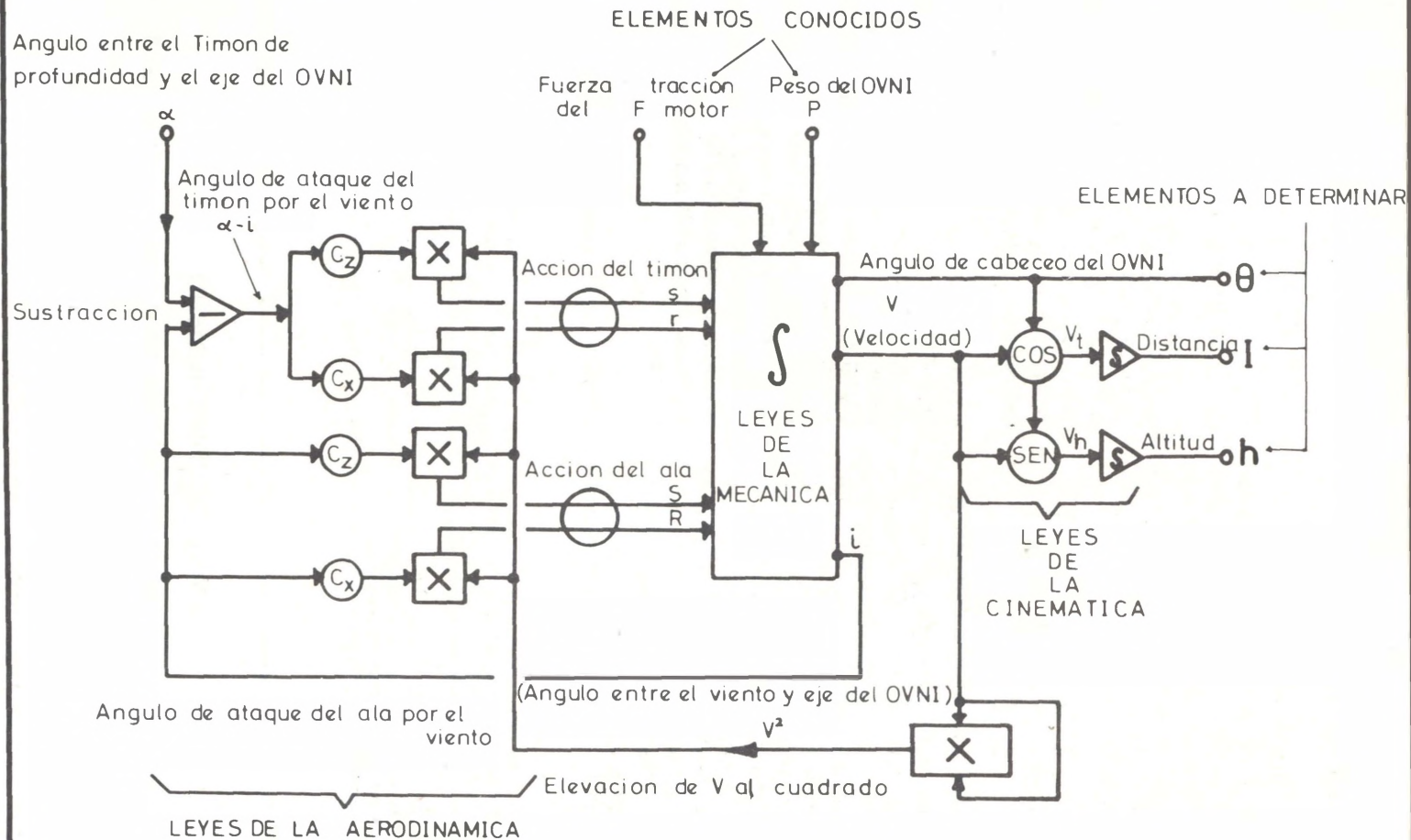
FIGURA 2. Diagrama funcional del conjunto de relaciones establecidas por las leyes de la física entre los elementos de un OVNI en vuelo en la atmósfera terrestre.
