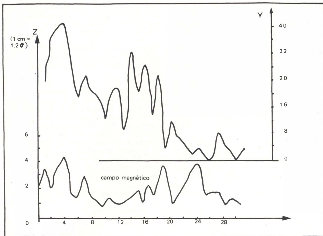
FIGURA 4. Gráfico comparativo de la distribución de observaciones de OVNI y las perturbaciones en la componente vertical del campo magnético terrestre, Chambon-la-Forêt, octubre 1954.
