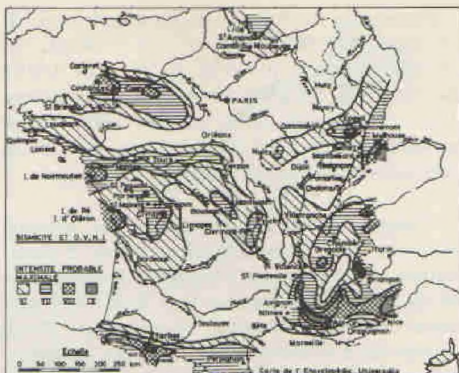
Carte de la France sismique (tirée de l'Encyclopédia Universalis).
