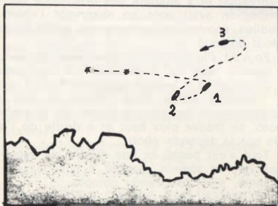
DIAGRAMME OBTENU APRES PROJECTION DES TROIS PHOTOS.
