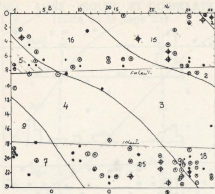
Fig 6 FEVRIER 1974 - ZONE NOIRE: 45 - ECLAIRCE 52
