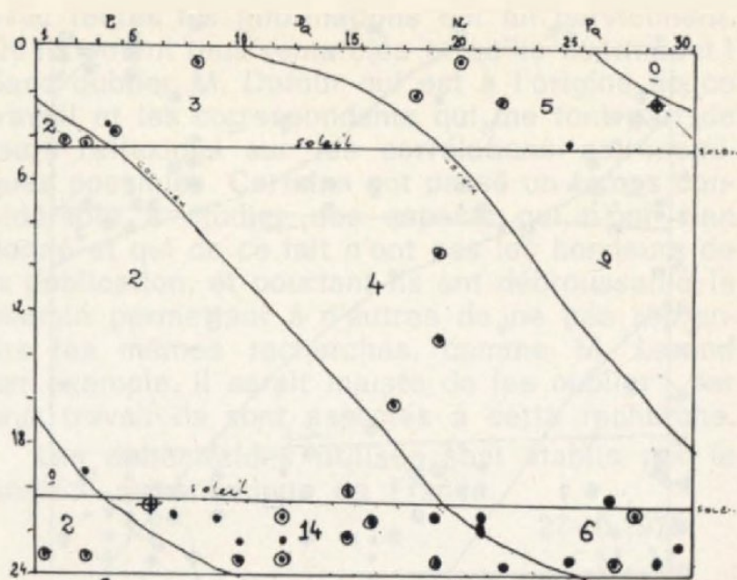
Fig 5. JUIN 1974 - ZONE NOIRE 21 - ZONE ECLAIRÉE 19
