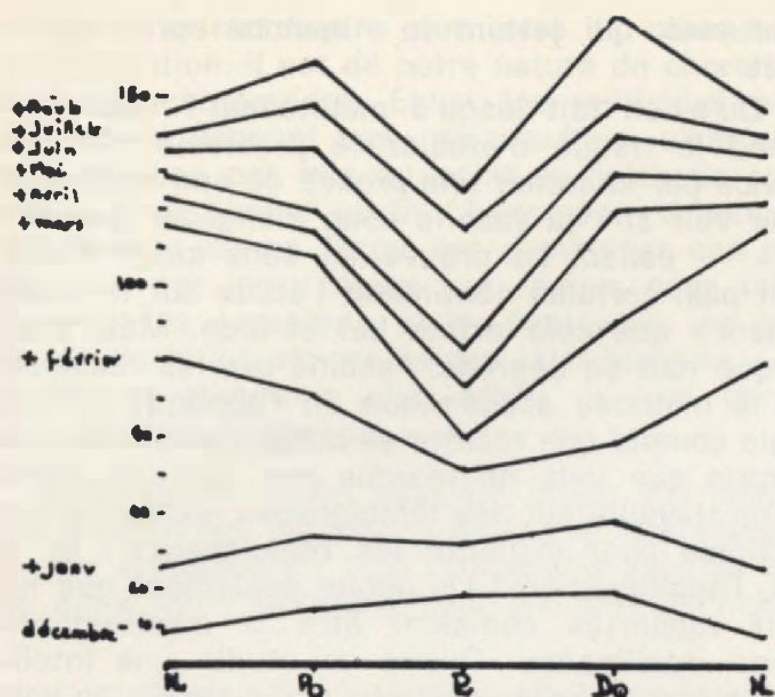
Fig 3. Observations et quartiers
