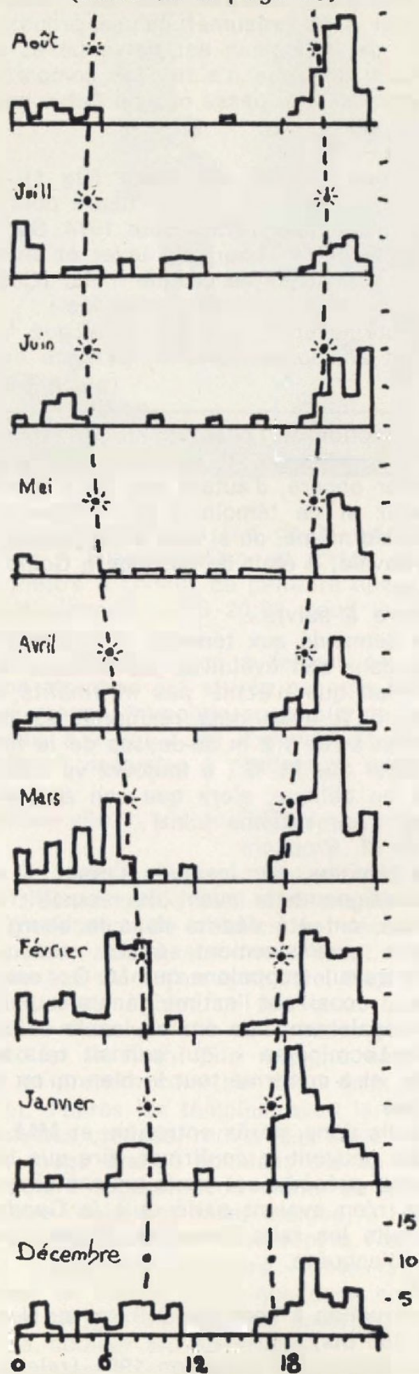
Fig. 1 : en fonction du Soleil
