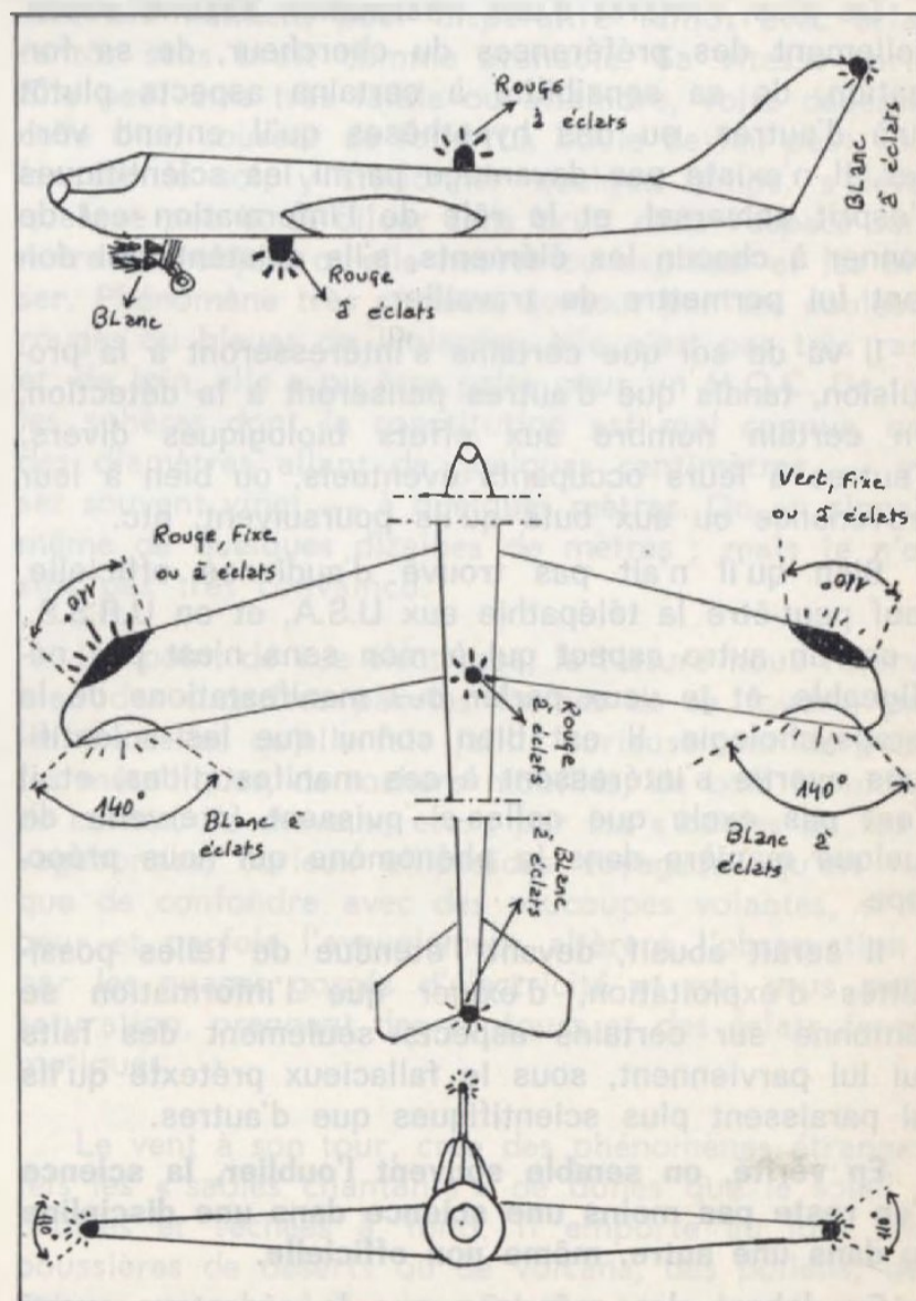
Dessin de J. DERACHE
