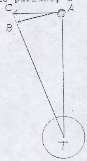
Fig. 131. Comment la Lune tombe vers la Terre, sans jamais la rencontrer. Si la Terre ne l'attirait pas, la Lune se déplacerait en ligne droite suivant A-C. L'attraction la fait tomber vers la Terre, de l'espace C-B, de telle manière que T-B reste égal à T-A.
